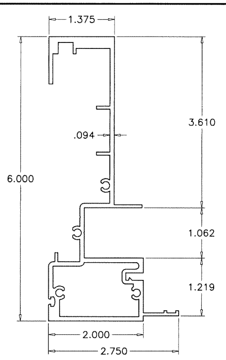
⑤ FRAME JAMB
