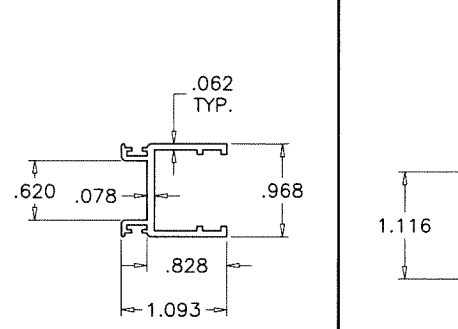
⑤ FRAME JAMB
